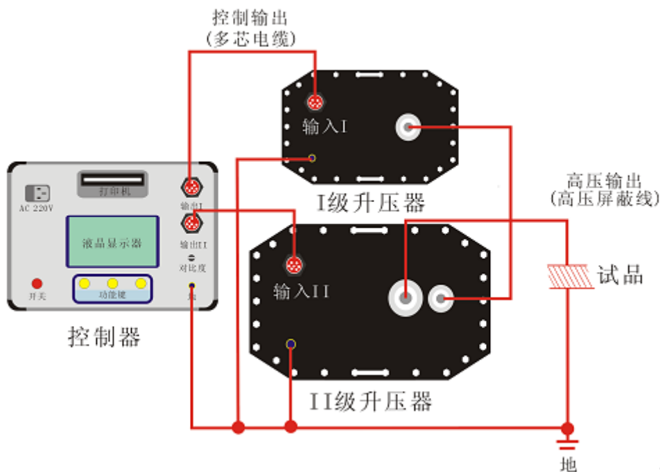
图 4 （连线图）
